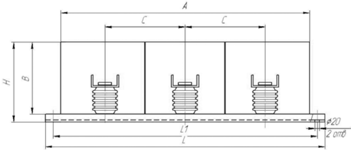
Рис. 9. Токопровод ТЗПР напряжением 10 кВ
