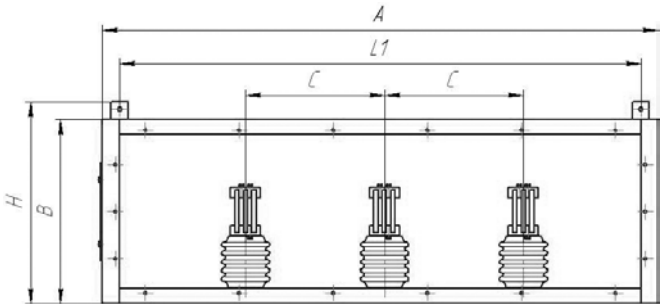
Рис. 11. Токопровод ТЗПР напряжением 10 кВ
