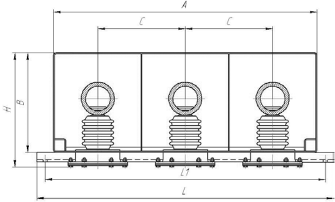
Рис. 9. Токопровод ТЗПР напряжением 10 кВ
