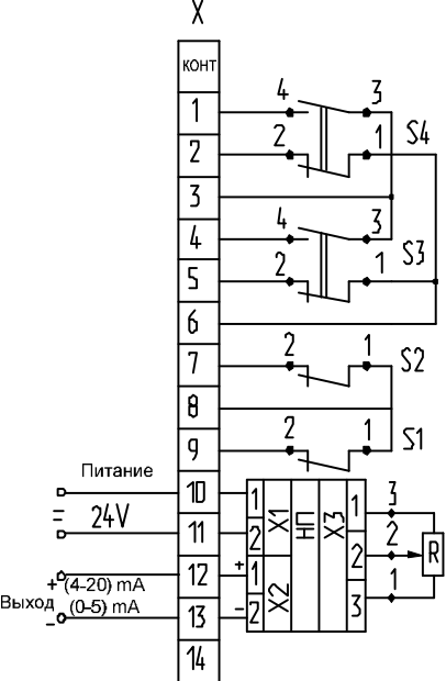
Рисунок А.4 -Схема электрическая принципиальная БСПТ исполнения ЯЛБИ.426449.088-16, -17
