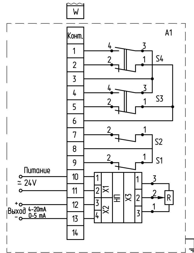
Рисунок Б.4- Схема электрическая принципиальная механизма с парным включением микровыключателей в БСПТ-ИВТ6 (поставляется по специальному заказу) Остальное см. рисунок Б.1
