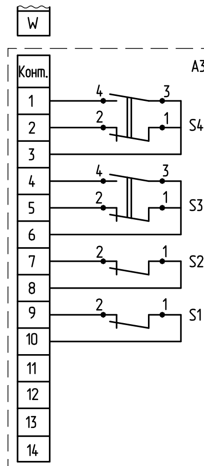
Рисунок Б.3- Схема электрическая принципиальная механизма с БСПМ-ИВТ6 Остальное см. рисунок Б.1
