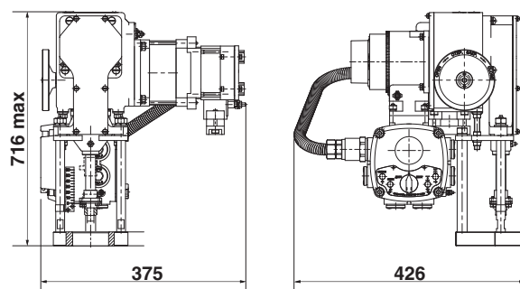
с блоком КИМ1 с ПМУ во взрывозащищенном исполнении
