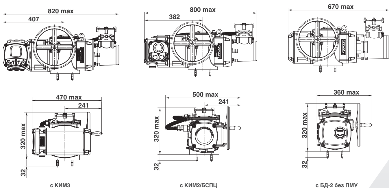
Габаритные размеры. Рисунок 3 (ПЭМ-Б250-12)
