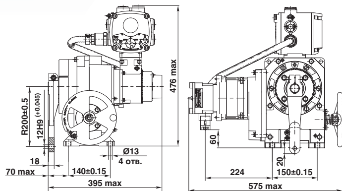
Рычажное исполнение (МЭО)
