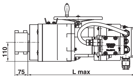
с КИМ2/БСПЦ
