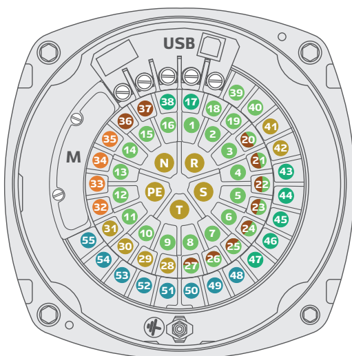
Клеммное винтовое подключение
