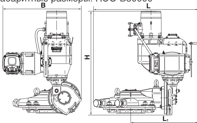
с КИМЗ
