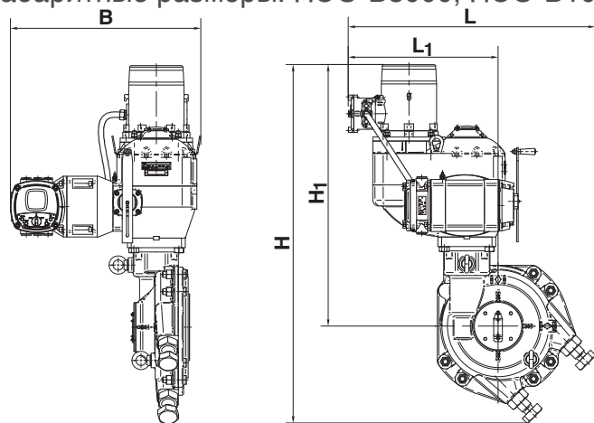
с КИМЗ
