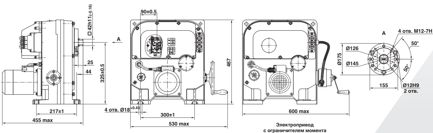
Габаритные размеры. Фланцевое исполнение. Рисунок Г
