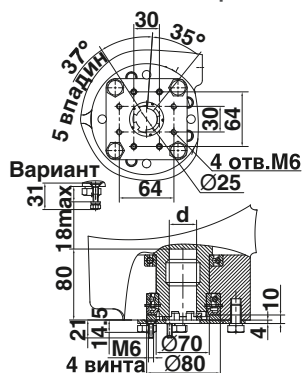
ПЭМ-М15-15, ПЭМ-М25-15
