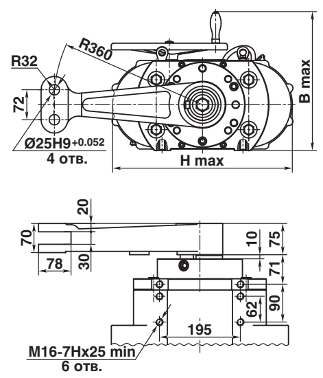
с БД-2 (БСПЦ) без ПМУ
