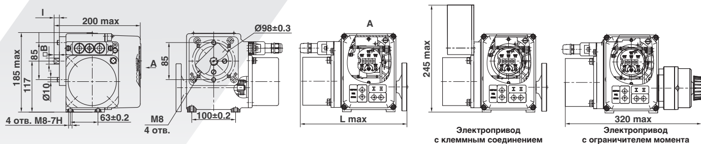
Габаритные размеры. Фланцевое исполнение. Рисунок А
