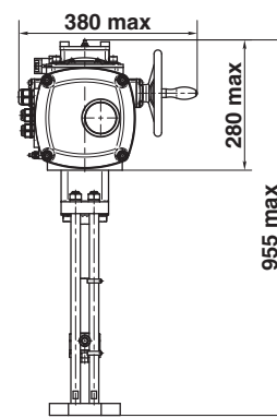
с БД-2 без ПМУ
