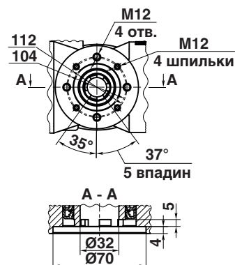
ПЭМ-А100-12
