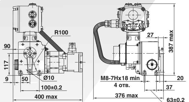
Рычажное исполнение (МЭО)
