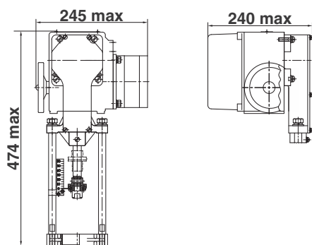
с блоком КИМ1 с ПМУ в общепромышленном исполнении
