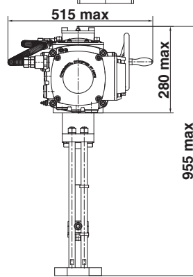
с КИМ2/БСПЦ
