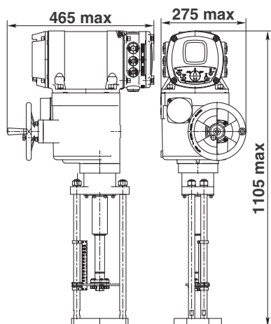
с КИМ3
