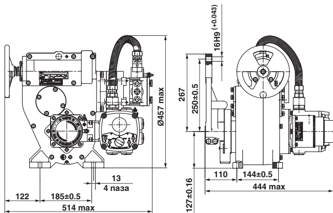
Рычажное исполнение (МЭО)
