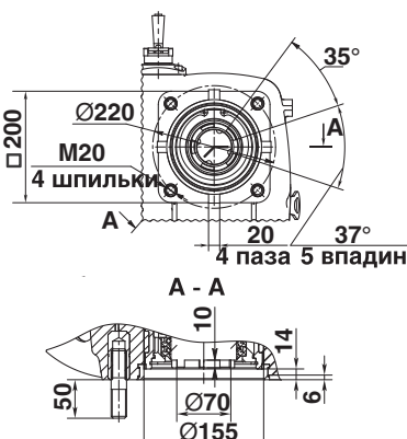
ПЭМ-В400-11, ПЭМ-В630-11, ПЭМ-В700-11, ПЭМ-В1000-11, ПЭМ-В1400-11, ПЭМ-В1500-11
