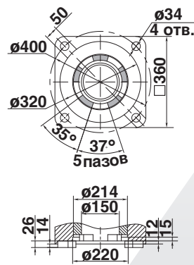
ПЭМ-Д5000-11М, ПЭМ-Д7500-11М, ПЭМ-Д9000-11М
