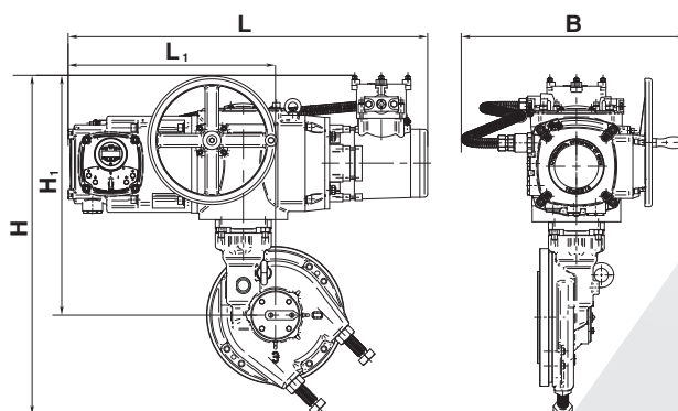
с КИМ2/БСПЦ
