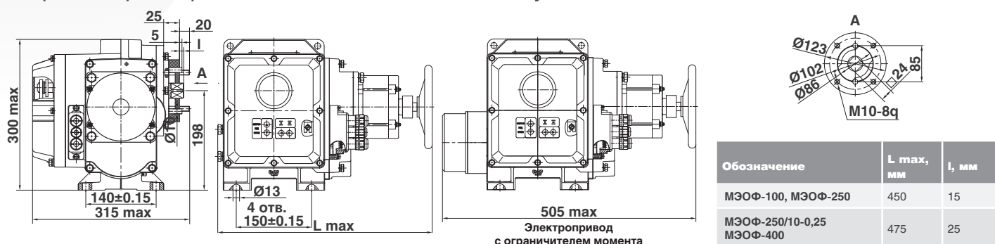
Габаритные размеры. Фланцевое исполнение. Рисунок Б
