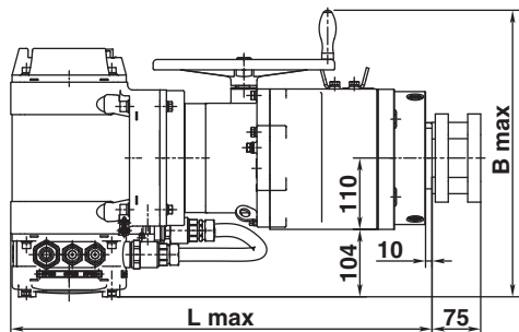
с КИМЗ
