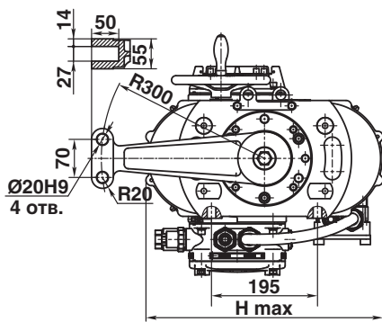
с КИМЗ
