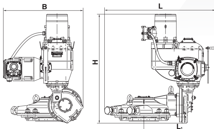
с КИМ2/БСПЦ
