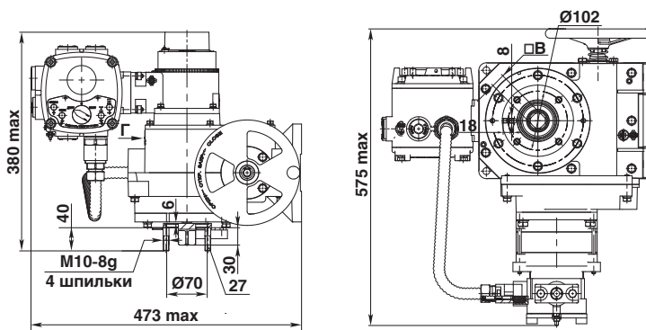
Фланцевое исполнение (МЭОФ)
