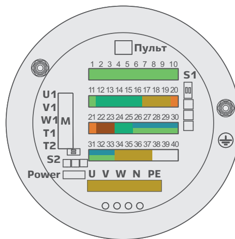
Разъемное (быстросъемное) подключение
