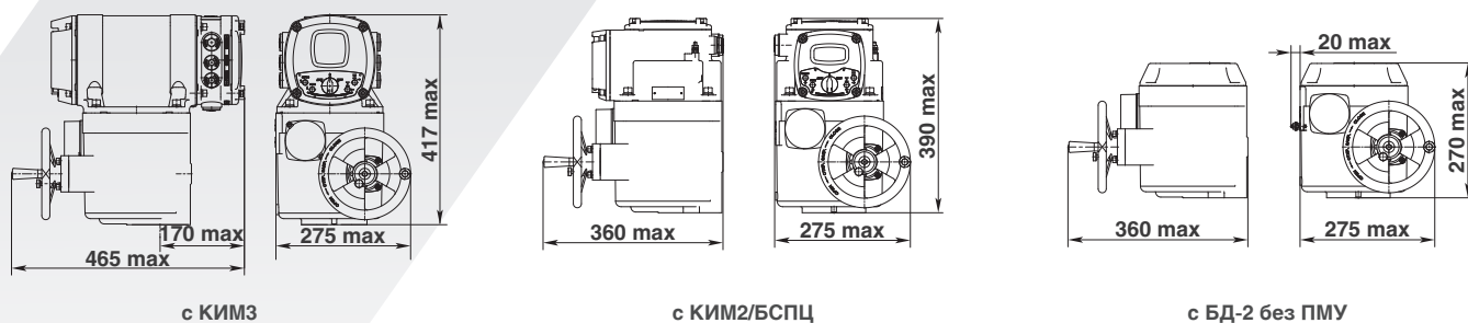
Габаритные размеры. Рисунок 2 (ПЭМ-А100-12)
