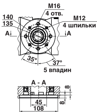
ПЭМ-Б250-12
