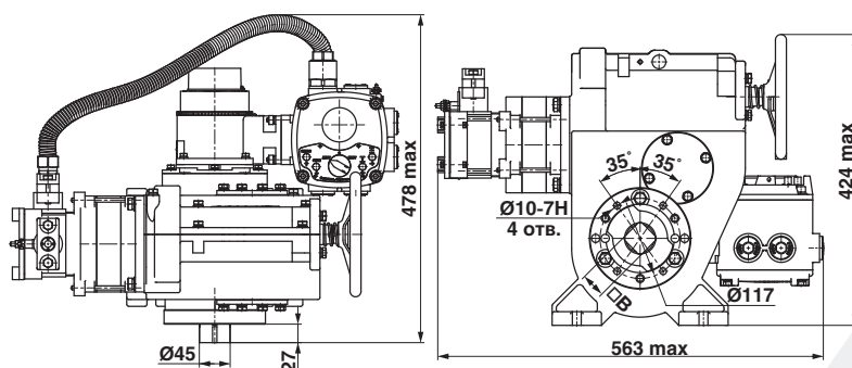
Фланцевое исполнение (МЭОФ)
