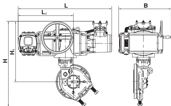
с КИМЗ
