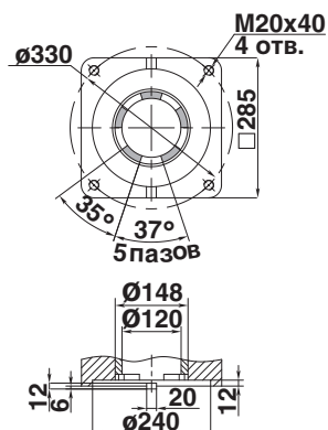
ПЭМ-Г2500-11М
