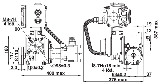
Фланцевое исполнение (МЭОФ)
