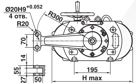
с БД-2 (БСПЦ) без ПМУ
