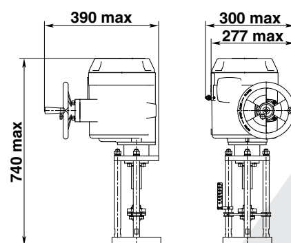
с БД-2 без ПМУ
