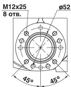
ПЭМ-А50-15, ПЭМ-А100-15
