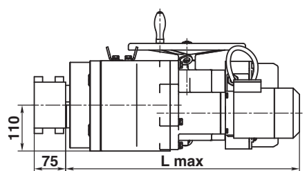
с БД-2 (БСПЦ) без ПМУ
