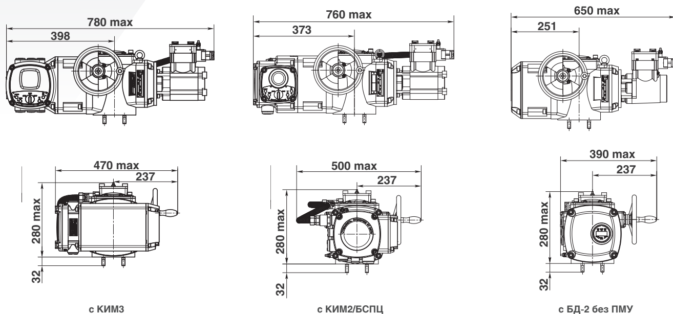
Габаритные размеры. Рисунок 2 (ПЭМ-А100-12)
