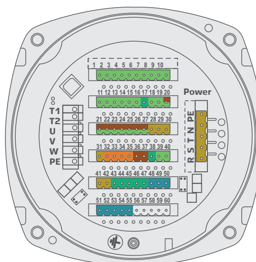
Разъемное (быстросъемное) подключение
