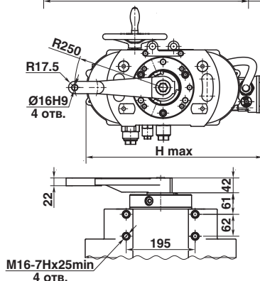
с КИМ2/БСПЦ
