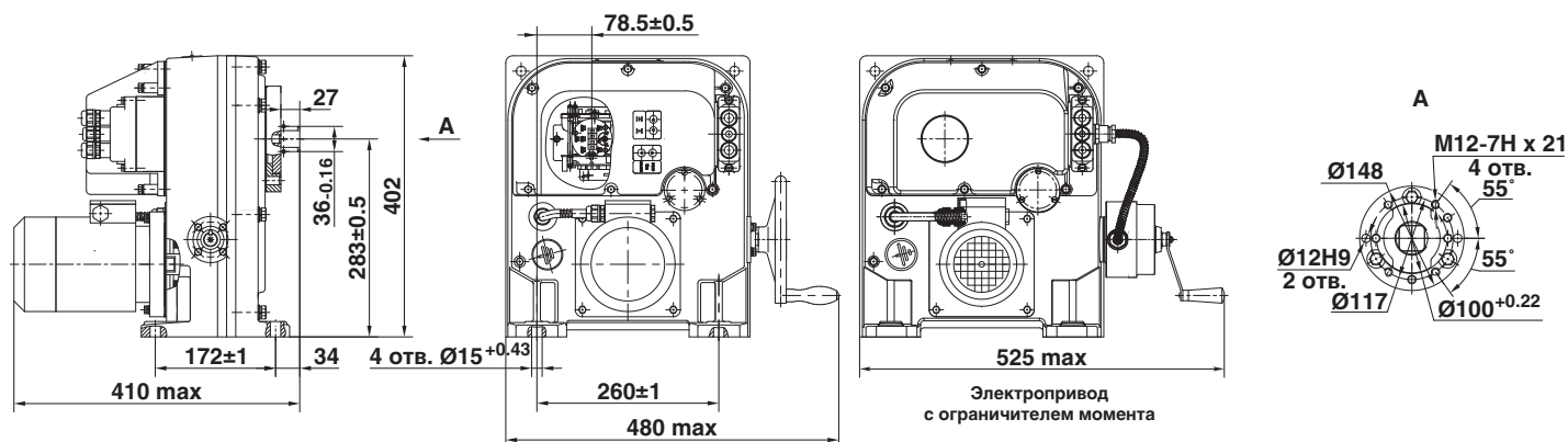
Габаритные размеры. Фланцевое исполнение. Рисунок В
